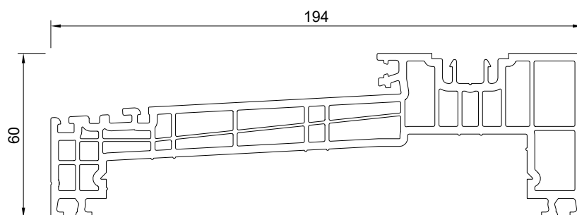
95200 - profil dolny - szary
