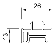
90209 - listwa szyny górnej - biała 95209 - listwa szyny górnej - szara
