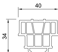
90202 - listwa dolna skrzydła
