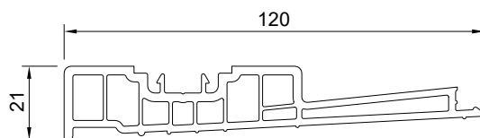
95201 - nakładka profilu dolnego - szary
