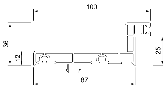
90203 - listwa uszczelniająca skrzydło
