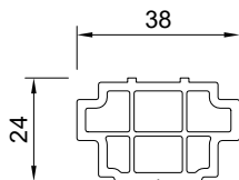
90206 - listwa ustalająca
