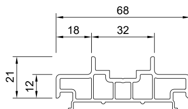
90205 - listwa uszczelniająca słupek ruchomy
