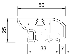
90208 - listwa zamykająca
