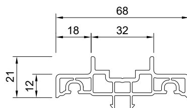
90204 - listwa uszczelniająca
